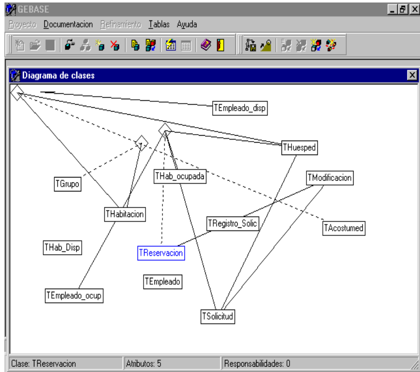
Diagrama de clases antes de aplicar el algoritmo.
