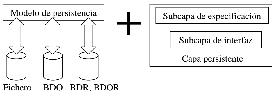
Figura 1. Estructura del método DIBAO.
