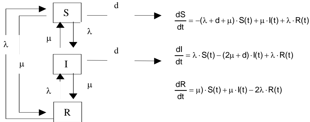
Figura 3. Modelo SIR.
